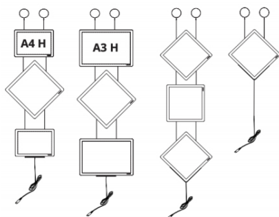
INSTALACJA Z VM START NOW DO MONTAŻU BEZPOŚREDNIO NA SZKLE
